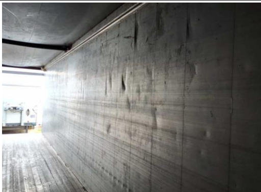
Wände Innenraum links und rechts verformt
