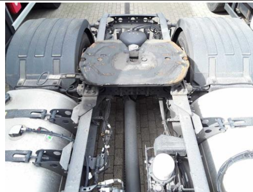
Ansicht Sattelplatte
