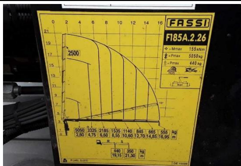
Ansicht Lastdiagramm
