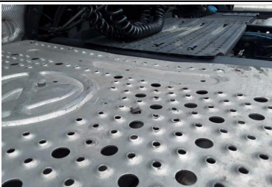
Hitzeschutz und Plattform verformt
