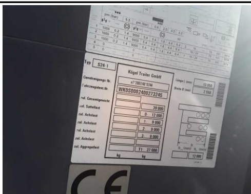
Ansicht Typenschild
