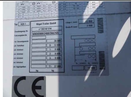
Ansicht Typschild
