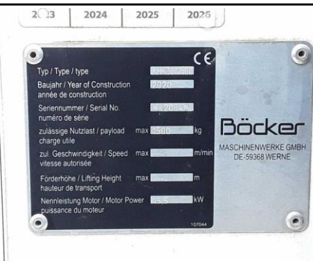
Ansicht Typschild
